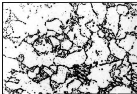
Балл 5, 500 x , электролитическое травление
