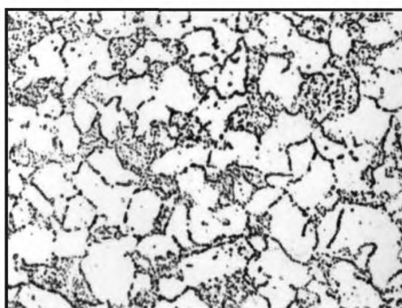
Балл 4, 500 x , электролитическое травление
