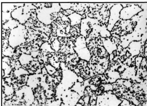
Балл 3, 500 x , электролитическое травление
