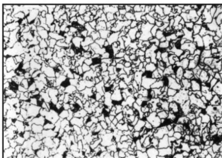
Балл 5, 100 \times
