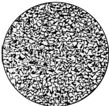
Балл 0
