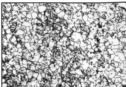
Балл 5, 100 x , химическое травление
