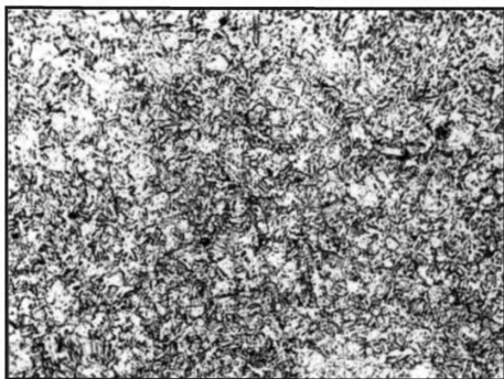
Балл 1, 100 x , химическое травление
