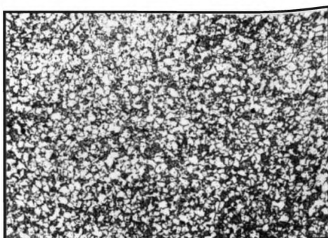
Балл 4, 100 x , электролитическое травление
