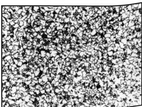
Балл 4, 100 x , химическое травление
