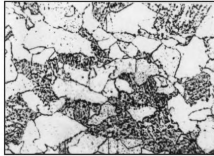
Балл 2, 500 ×
