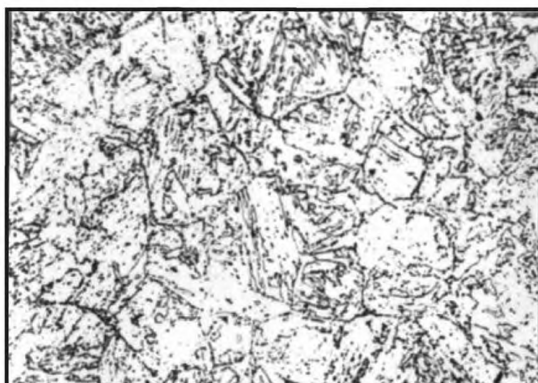
Балл 1, 100 x
