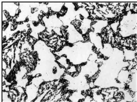
Балл 8, 500 x , химическое травление
