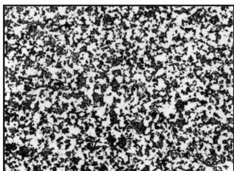
Балл 8, 100 x , химическое травление
