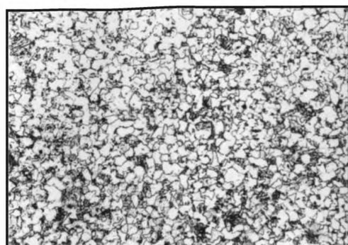
Балл 6, 100 x , химическое травление
