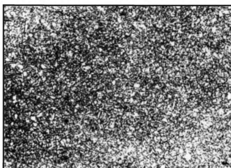
Балл 1, 100 x , электролитическое травление
