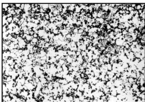
Балл 8, 100 x , электролитическое травление
