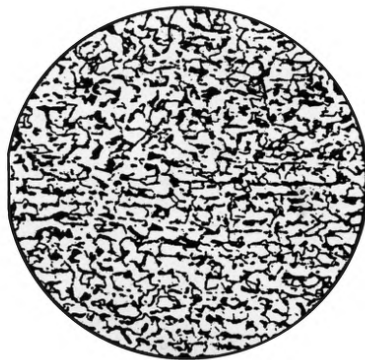
Балл 1
