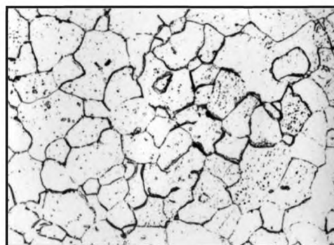
Балл 7, 500 x , химическое травление
