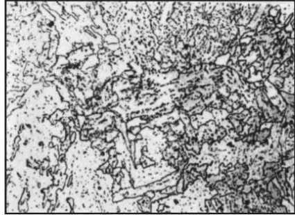
Балл 1, 500 ×
