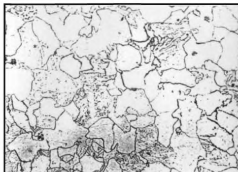
Балл 6, 500 x , химическое травление
