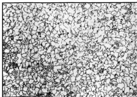
Балл 7, 100 x , химическое травление
