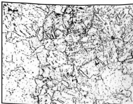
Балл 1, 500 x , химическое травление
