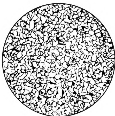
Балл 0
