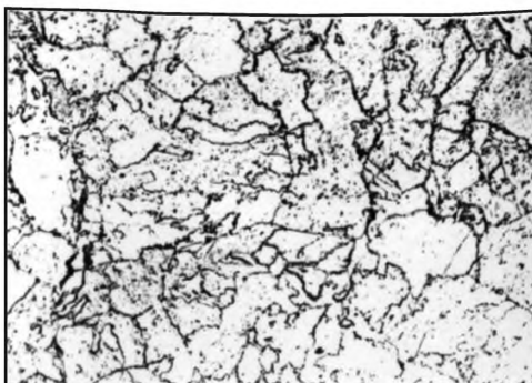
Балл 2, 500 x , химическое травление
