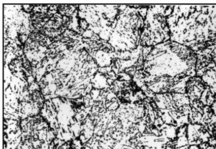
Балл 8, 100 x
