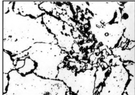
Балл 9, 500 x
