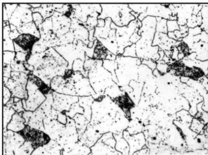
Балл 6, 100 x
