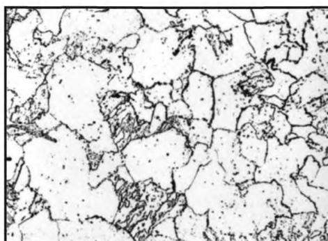
Балл 5, 500 x , химическое травление
