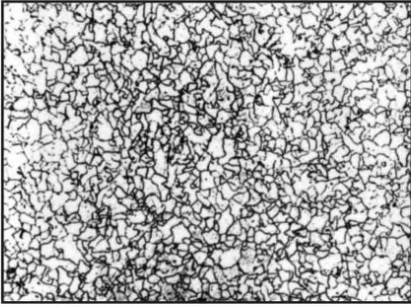
Балл 7, 100 x
